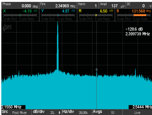
FFT display
