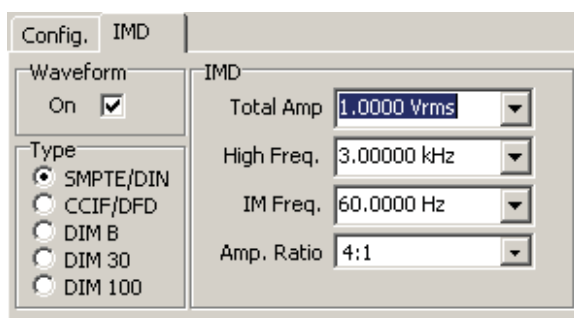
IMD Tab for SMPTE/DIN
